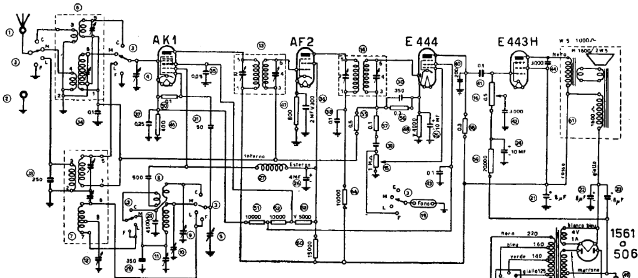
GELOSO. — Mod. G. 54. — Medie, corte e lunghe. — Media frequenza: 348 kHz. — Produzione: 1935-1936. (Tensioni anodiche: 238 V; entrata filtro: 340 V).
