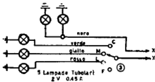
GELOSO. — Mod. G. 54. — Medie, corte e lunghe. — Media frequenza: 348 kHz. — Produzione: 1935-1936. (Tensioni anodiche: 238 V; entrata filtro: 340 V).
